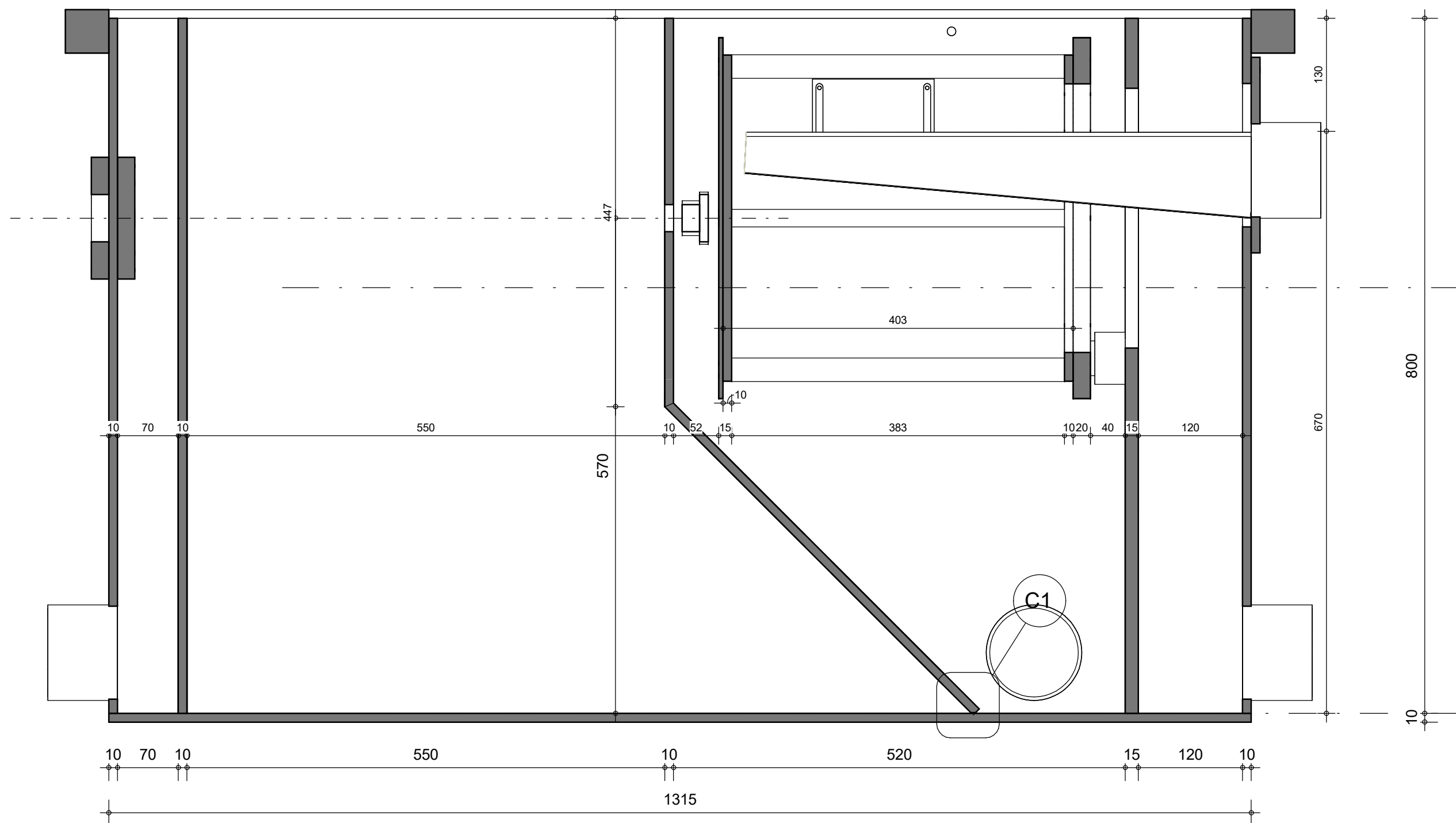
Doorsnede C 1:5
